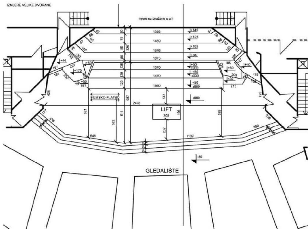
POZORNICA – IZMJERE STAGE – DIMENSIONS
