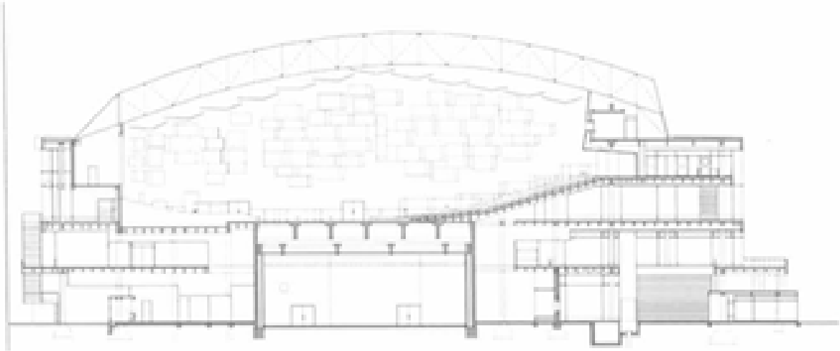
POZORNICA – IZMJERE STAGE – DIMENSIONS
